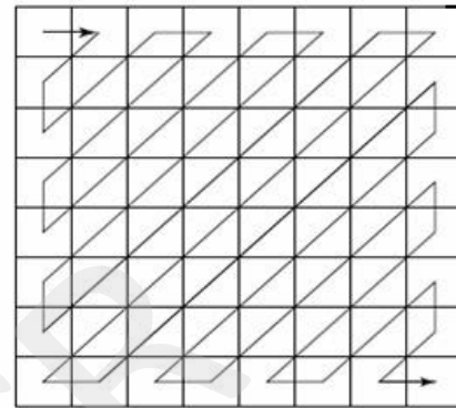
Figure4: Zig-Zag Reordering
